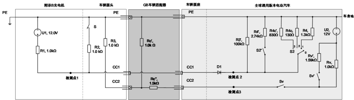
d) 连接至附录 B 充电机
