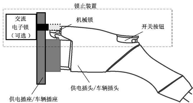
图 I.1 交流充电接口锁止装置(电流小于 16 A)示意图
