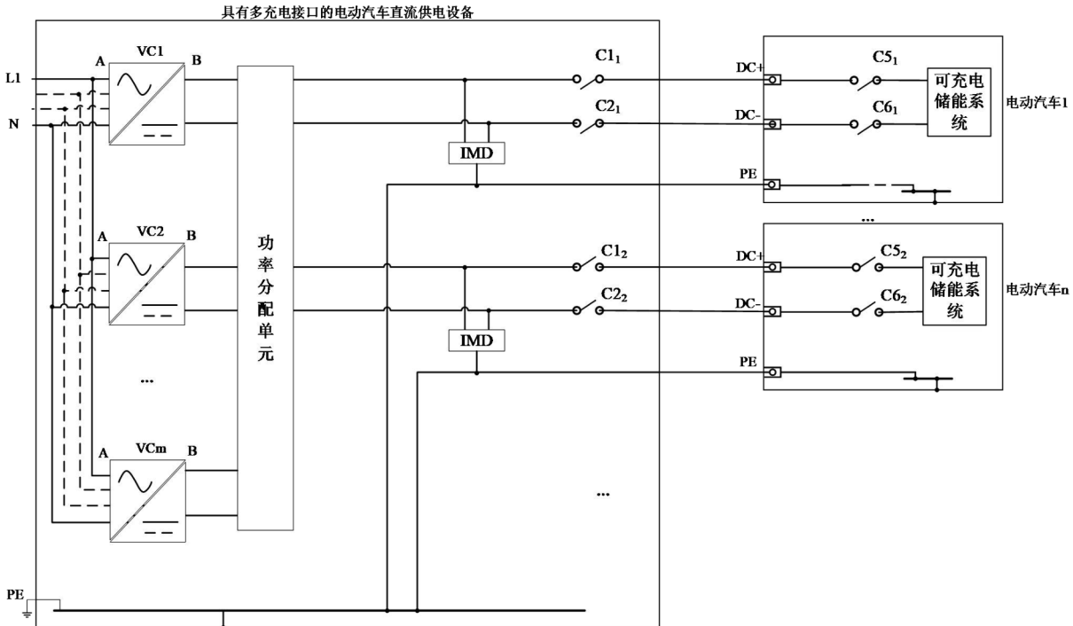
a) 不同时充电工作方式
